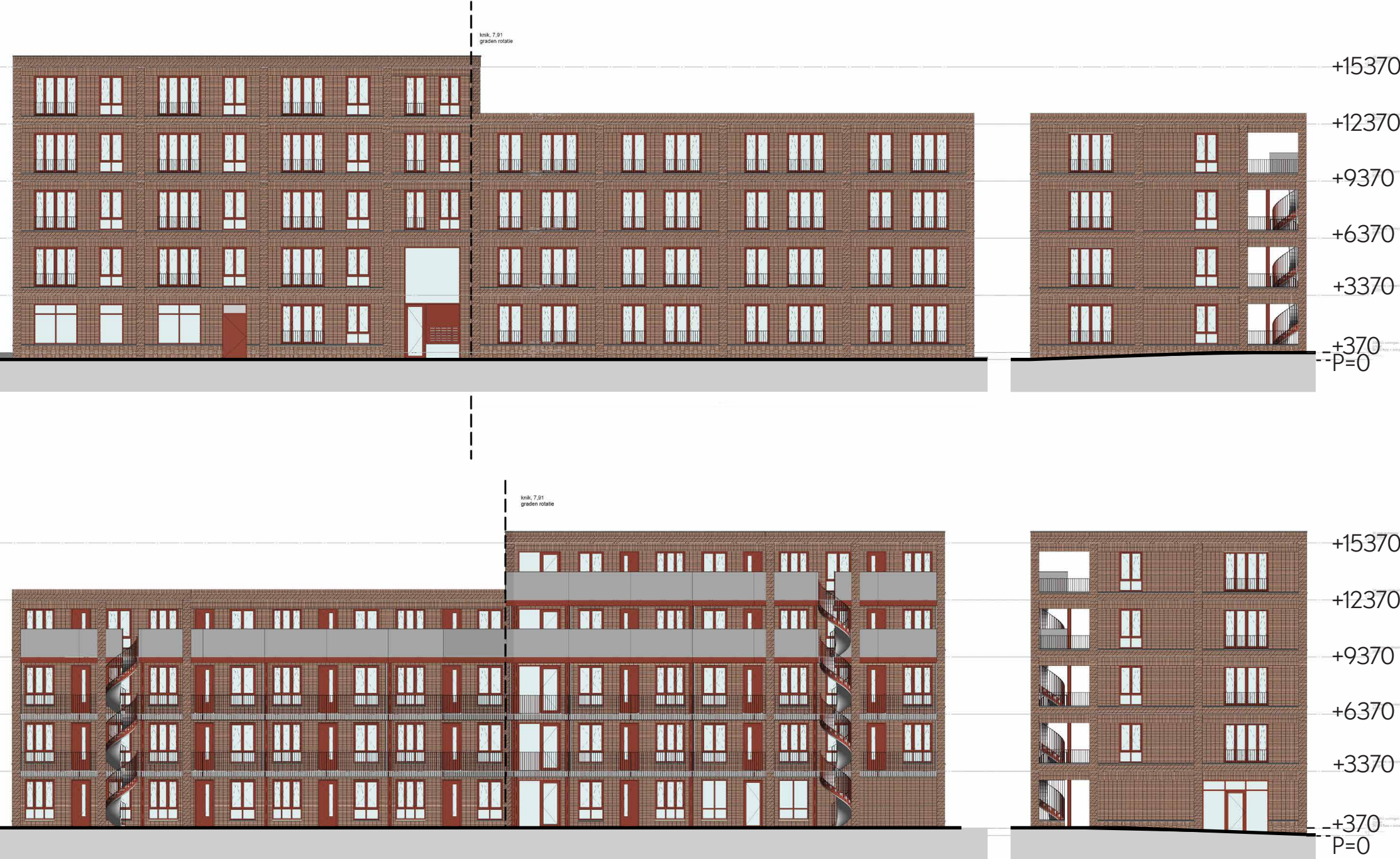
Gevelaanzichten
