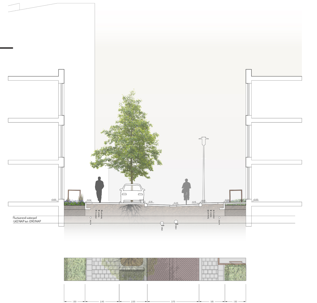
Doorsnede van de regentuin
