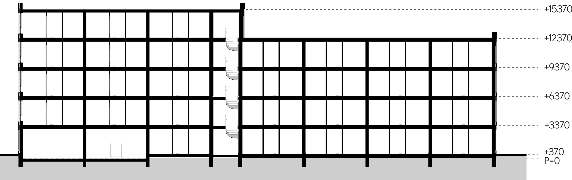
Doorsnede (1:200)
