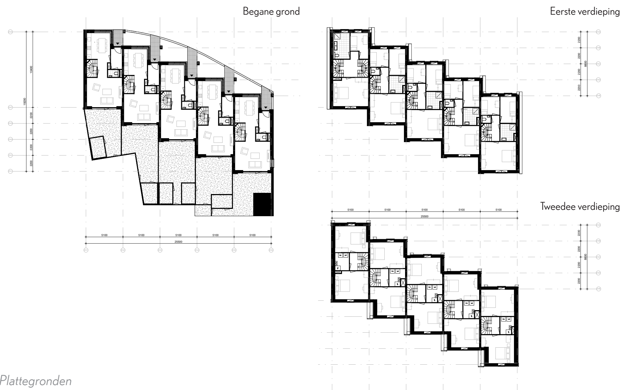
Plattegronden
