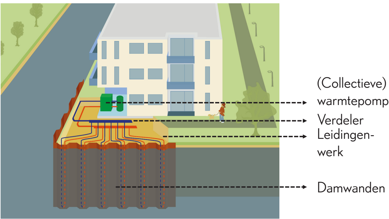
Werking Energiedamwand
